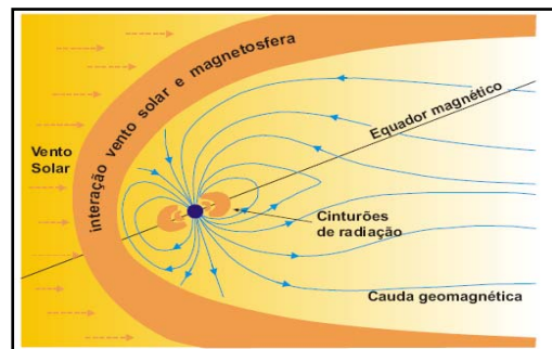
Figura 2. O vento solar interagindo com a Magnetosfera. Fonte: Teixeira et al , 2000.
