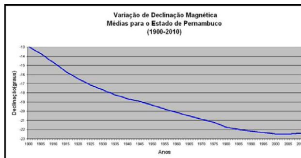
Figura 18. Gráfico da Declinação Magnética (D) (período de 1900 a 2010), pelo autor, com o modelo IGRF10, 2007.
