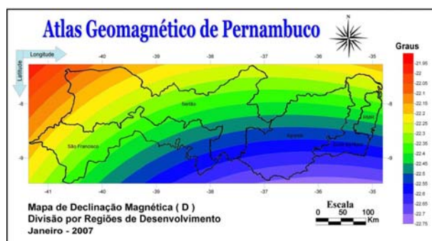
Figura 13. Mapa de Declinação Magnética (D) para o Estado de Pernambuco, construído pelo autor, 2007.
