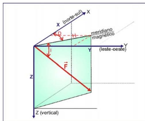
Figura 4. Componentes do Campo Magnético Terrestre. Fonte: Teixeira et al , 2000.
