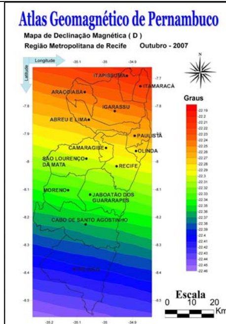
Figura 15. Mapa da Declinação Magnética (D) da Região Metropolitana de Recife, pelo autor, 2007.
