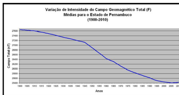
Figura 17. Gráfico do Campo Total de Pernambuco (período de 1900 a 2010), pelo autor, com o modelo IGRF10, 2007.
