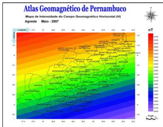
Figura 16. Mapa de Intensidade do Campo Geomagnético Horizontal (H) para o Agreste de Pernambuco, pelo autor, 2007.
