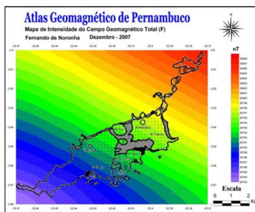
Figura 14. Mapa de Intensidade do Campo Geomagnético Total (F), para Fernando de Noronha, pelo autor, 2007.
