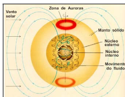
Figura 1. Movimentos do núcleo da Terra geram o campo magnético na superfície. Fonte: Teixeira et al , 2000.
